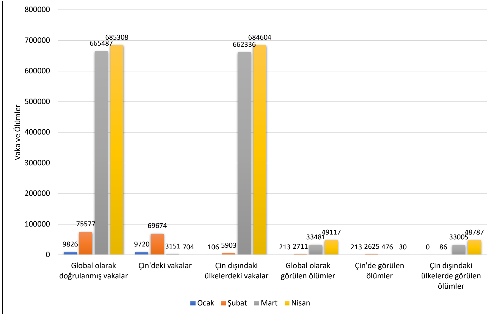
Tespit Edilen COVID-19 Toplam Vaka ve Ölümünün Aylara Göre Dağılım Grafiği, 31 Aralık 2019-09 Nisan 2020.
