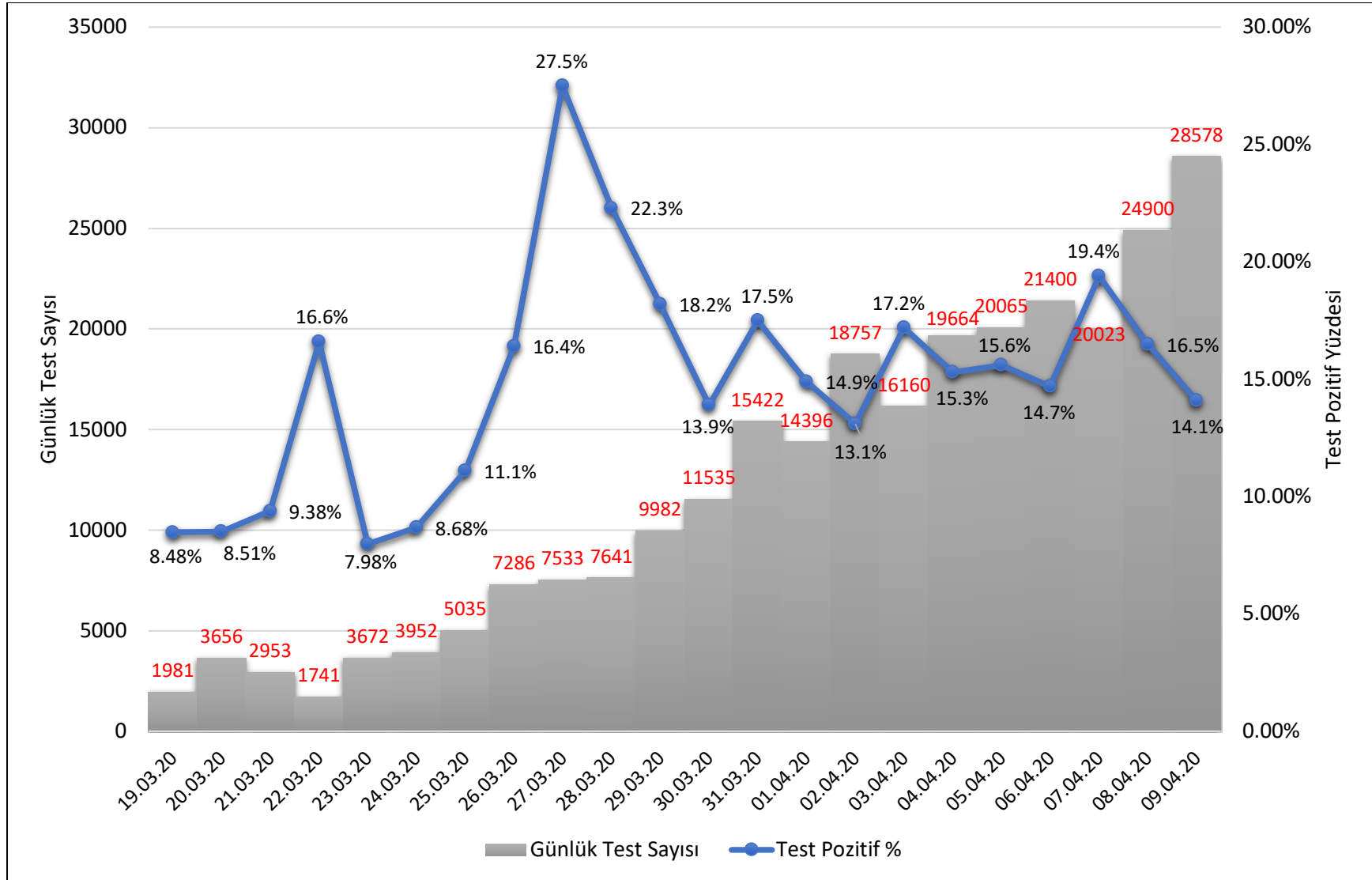
Türkiye’de COVID-19 Teşhisi Amacıyla Yapılan Günlük Test Sayısı ve Pozitif Yüzdesi Grafiği, 19 Mart-09 Nisan 2020. (Kaynak: Sağlık Bakanlığı)
