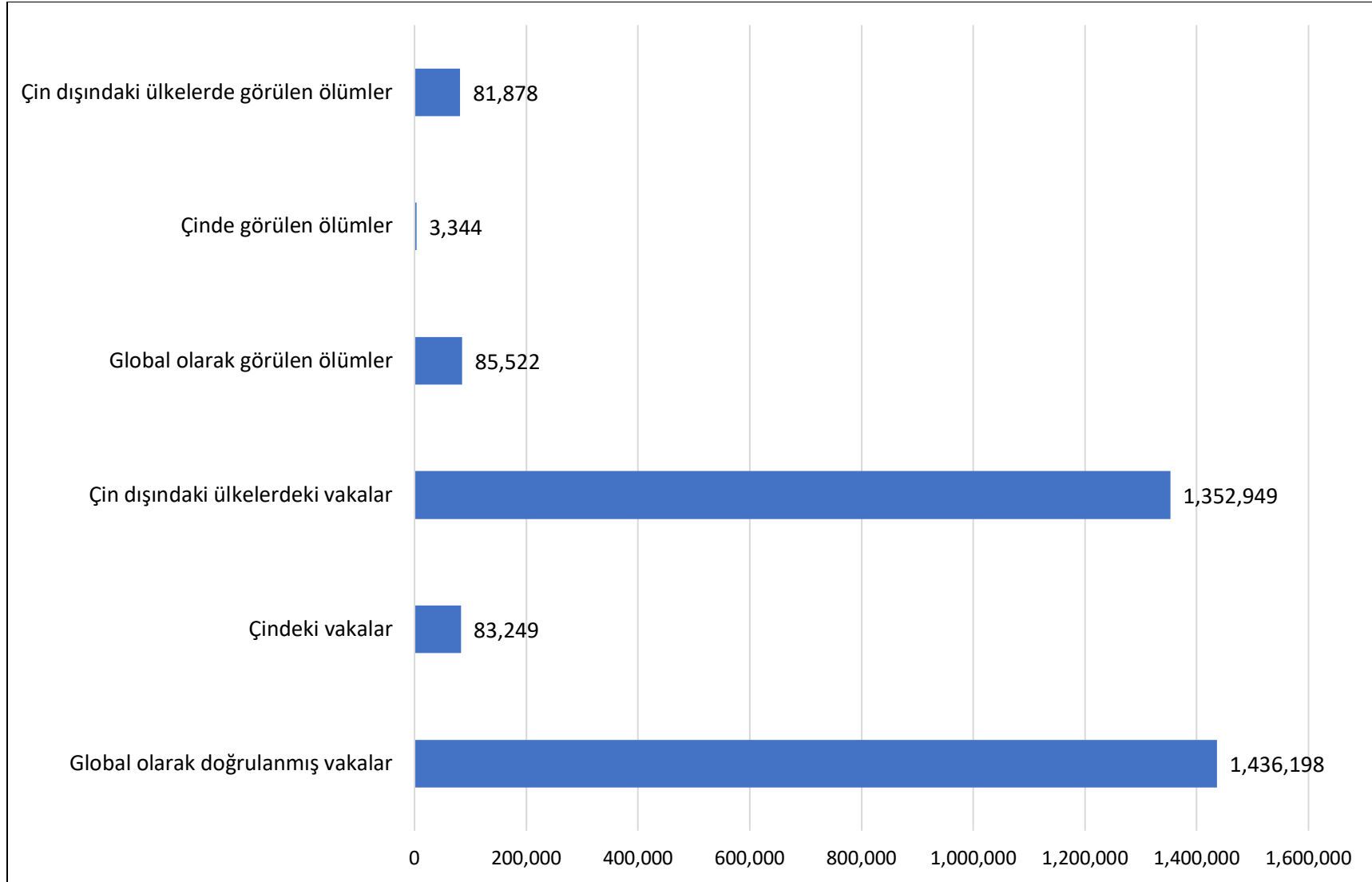
Çin ve Çin Dışındaki Ülkelerde Tespit Edilen COVID-19 Vaka ve Ölüm Grafiği, 31 Aralık 2019-09 Nisan 2020.
