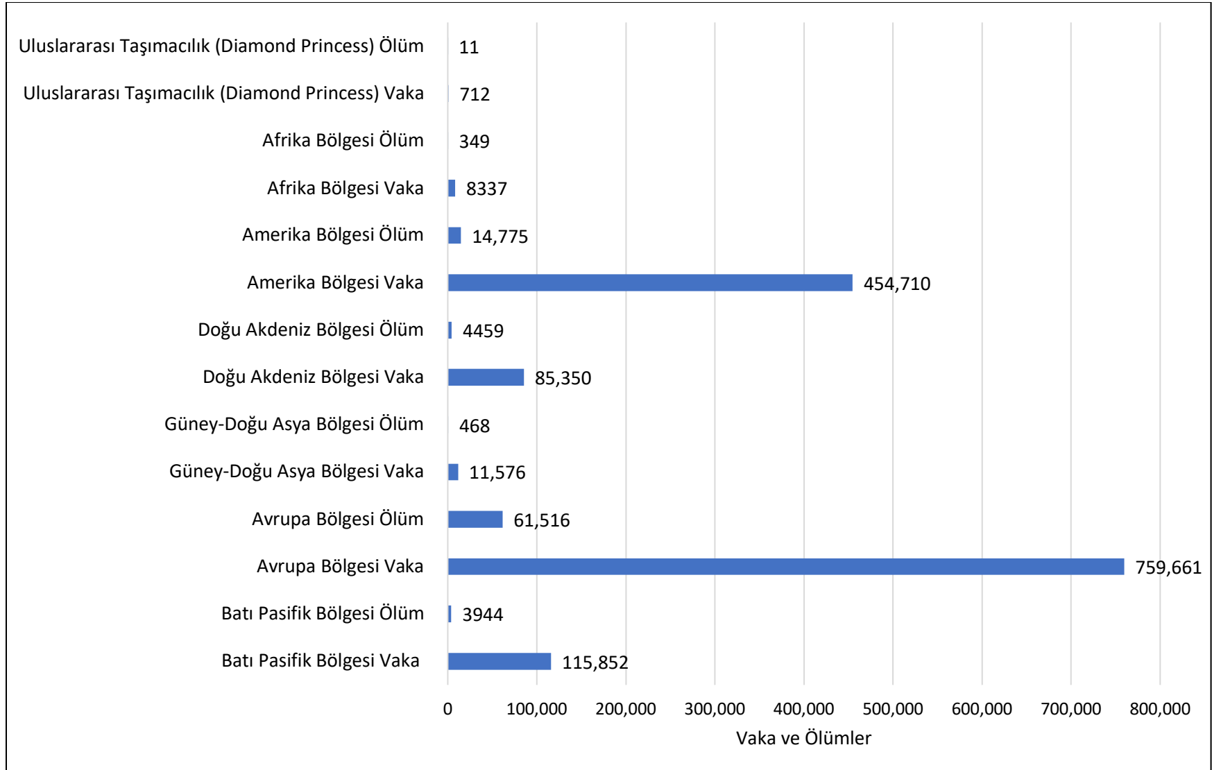
Global Olarak Bölgelerde Tespit Edilen COVID-19 Toplam Vaka ve Ölüm Sayıları Grafiği, 31 Aralık 2019-09 Nisan 2020.
