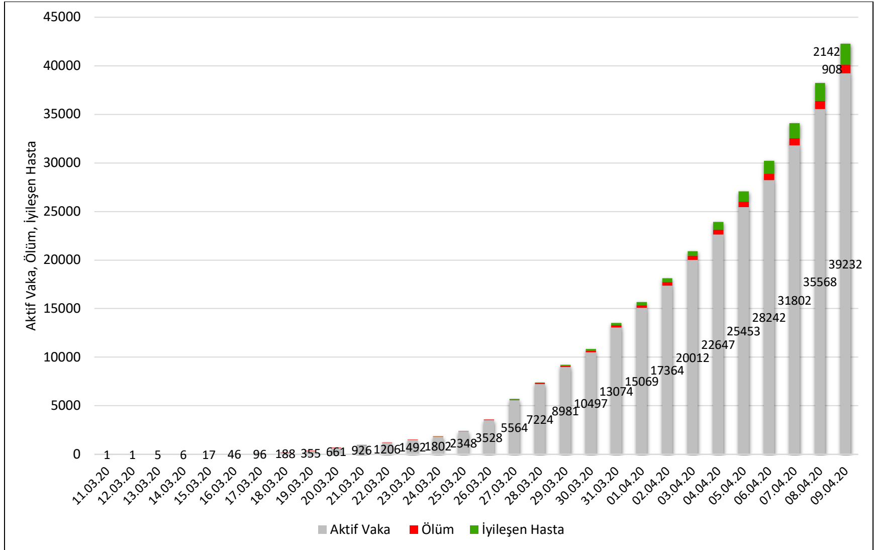
Türkiye’de COVID-19 Aktif Vaka, Ölüm ve İyileşen Hastaların Günlere Göre Dağılım Grafiği, 11 Mart-09 Nisan 2020. (Kaynak: Sağlık Bakanlığı)
