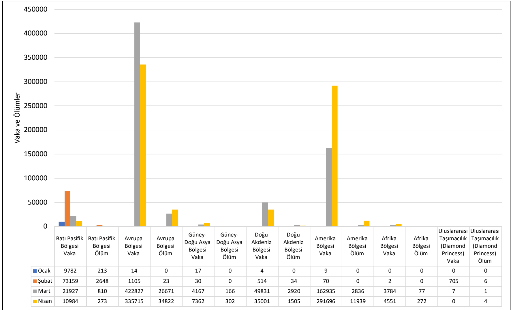
Global Olarak Bölgelerde Tespit Edilen COVID-19 Toplam Vaka ve Ölüm Sayılarının Aylara Göre Dağılım Grafiği, 31 Aralık 2019-09 Nisan 2020.
