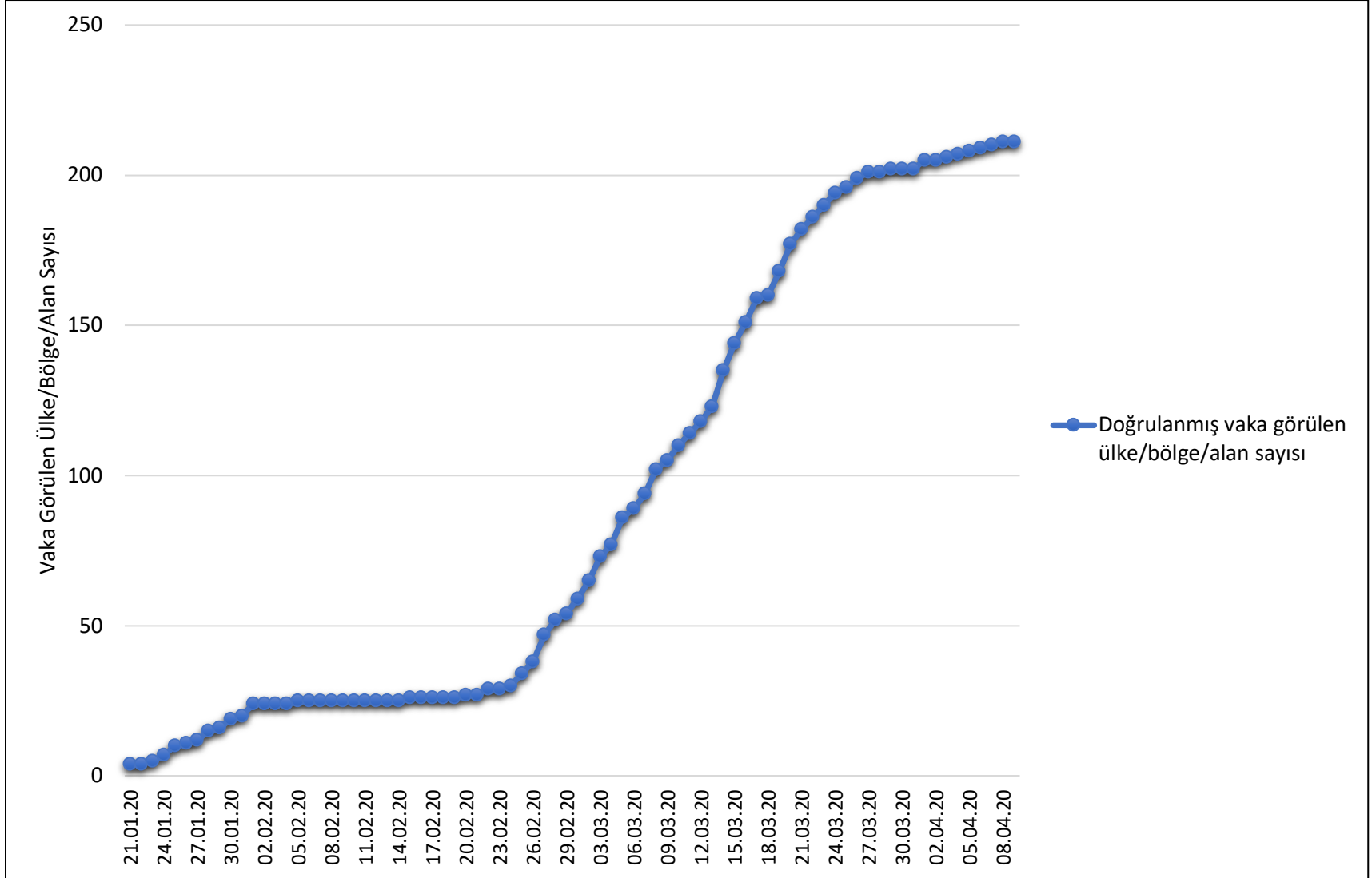
Doğrulanmış COVID-19 Vakası Görülen Ülke/Bölge/Alan Sayısı Grafiği, 31 Aralık 2019-09 Nisan 2020.
