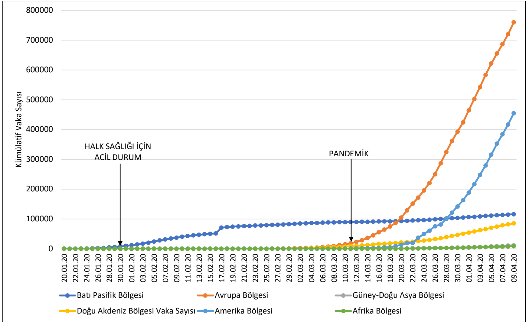
Global Olarak Bölgelerde Tespit Edilen COVID-19 Kümülatif Vaka Sayılarının Günlere Göre Dağılım Grafiği, 31 Aralık 2019-09 Nisan 2020.
