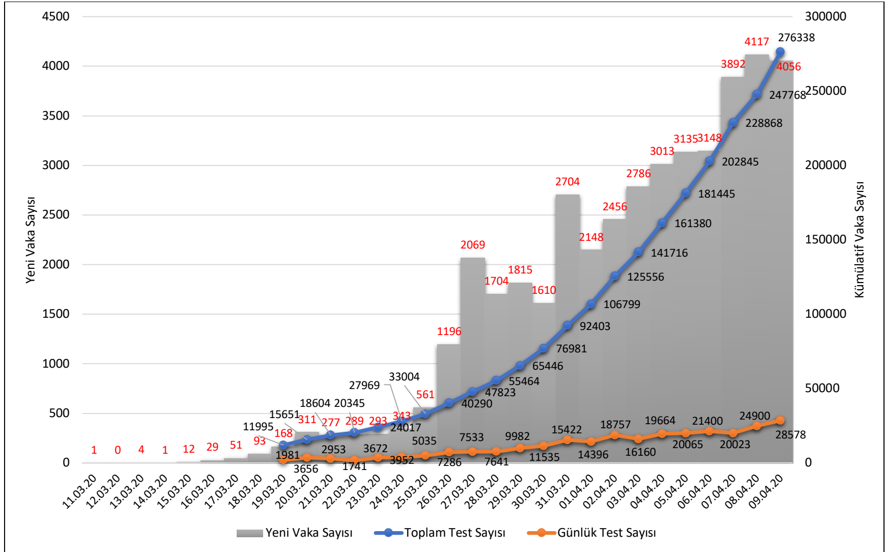
Türkiye’de COVID-19 Teşhisi Amacıyla Yapılan Toplam Test Sayısı, Günlük Test Sayısı ve Yeni Vaka Sayısı Grafiği, 11 Mart-09 Nisan 2020.
