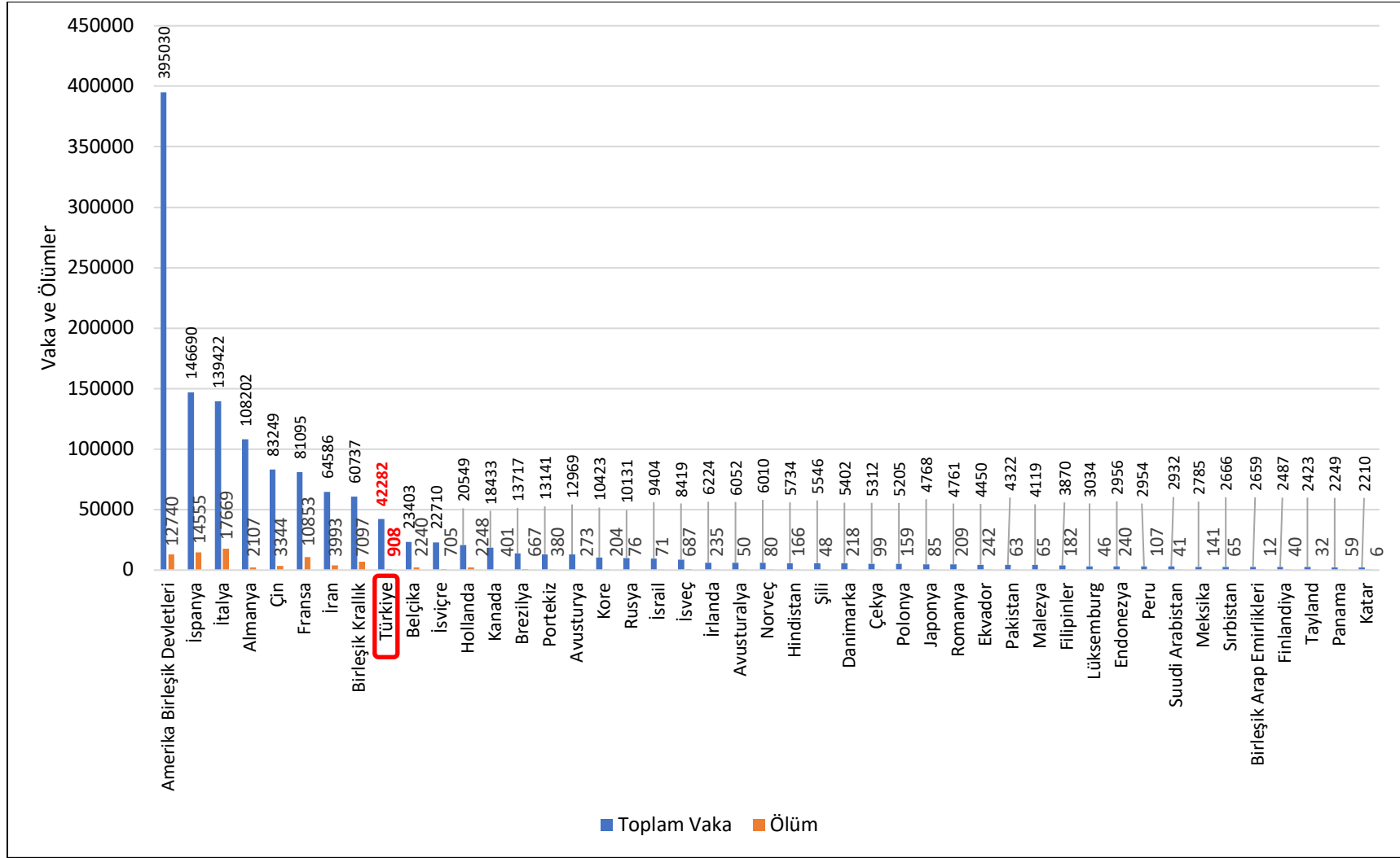
Tespit Edilen 2000'den Fazla COVID-19 Toplam Vaka ve Ölümlerin Ülkeler Düzeyinde Karşılaştırılma Grafiği, 31 Aralık 2019-09 Nisan 2020.
