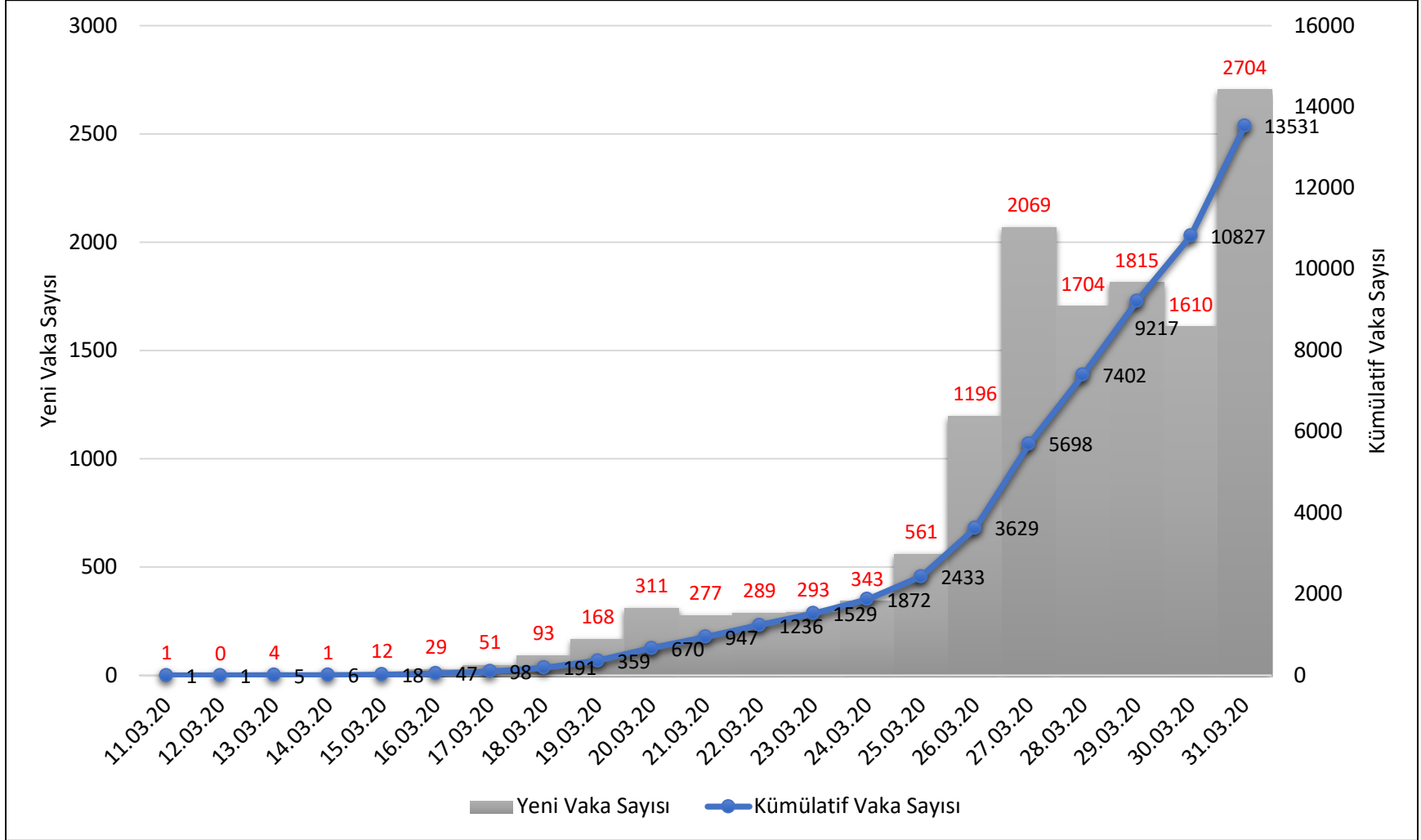
Türkiye’de Tespit Edilen COVID-19 Yeni Vakaların Epidemik Eğrisi, 11-31 Mart 2020.
