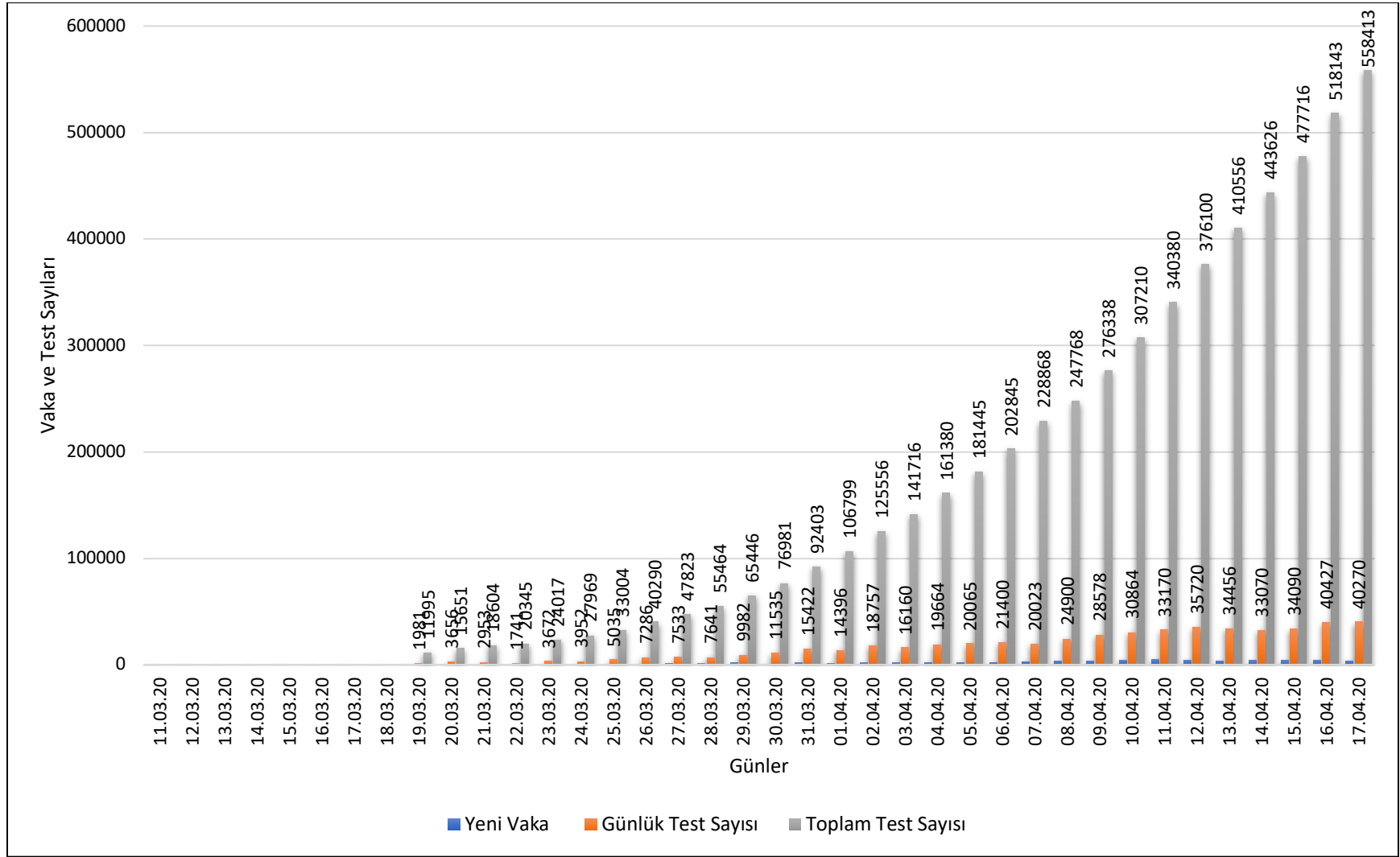
Türkiye’de COVID-19 Teşhisi Amacıyla Yapılan Toplam Test Sayısı, Günlük Test Sayısı ve Yeni Vaka Sayısı Grafiği, 11 Mart-17 Nisan 2020.
